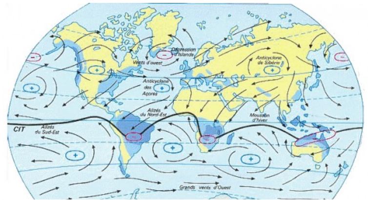
Doc 2 : Les principaux vents à la surface des océans.
